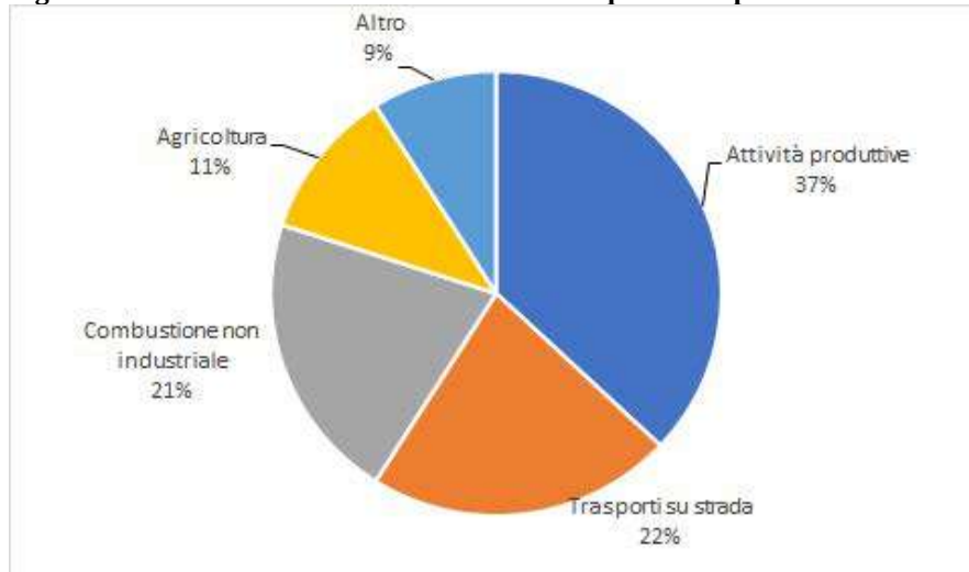
Figura 6.5 - Distribuzione di emissioni di CO 2 equivalente per macrosettore. Veneto - Anno 2017
