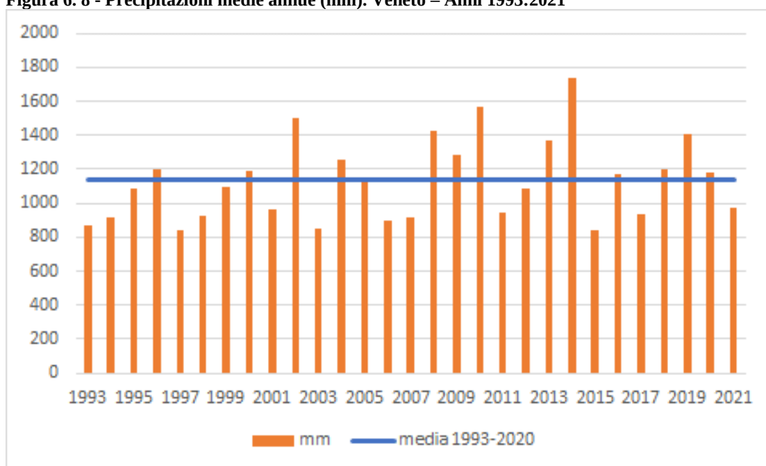
Figura 6. 8 - Precipitazioni medie annue (mm). Veneto – Anni 1993:2021
